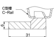
组装图 Shown assembled
