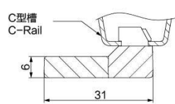
组装图 Shown assembled
